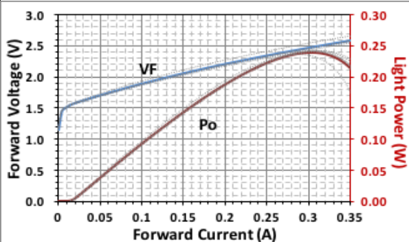
LIV Curve
